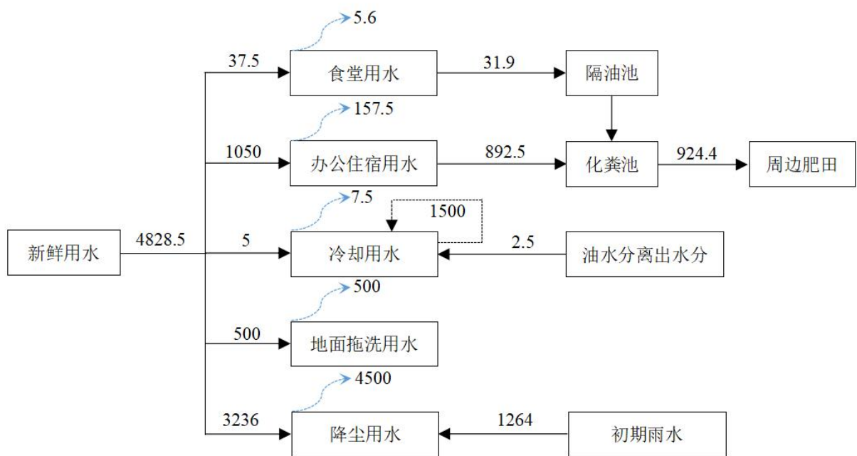
图2-1 水平衡图（单位： \text{m}^3/\text{a} ）
