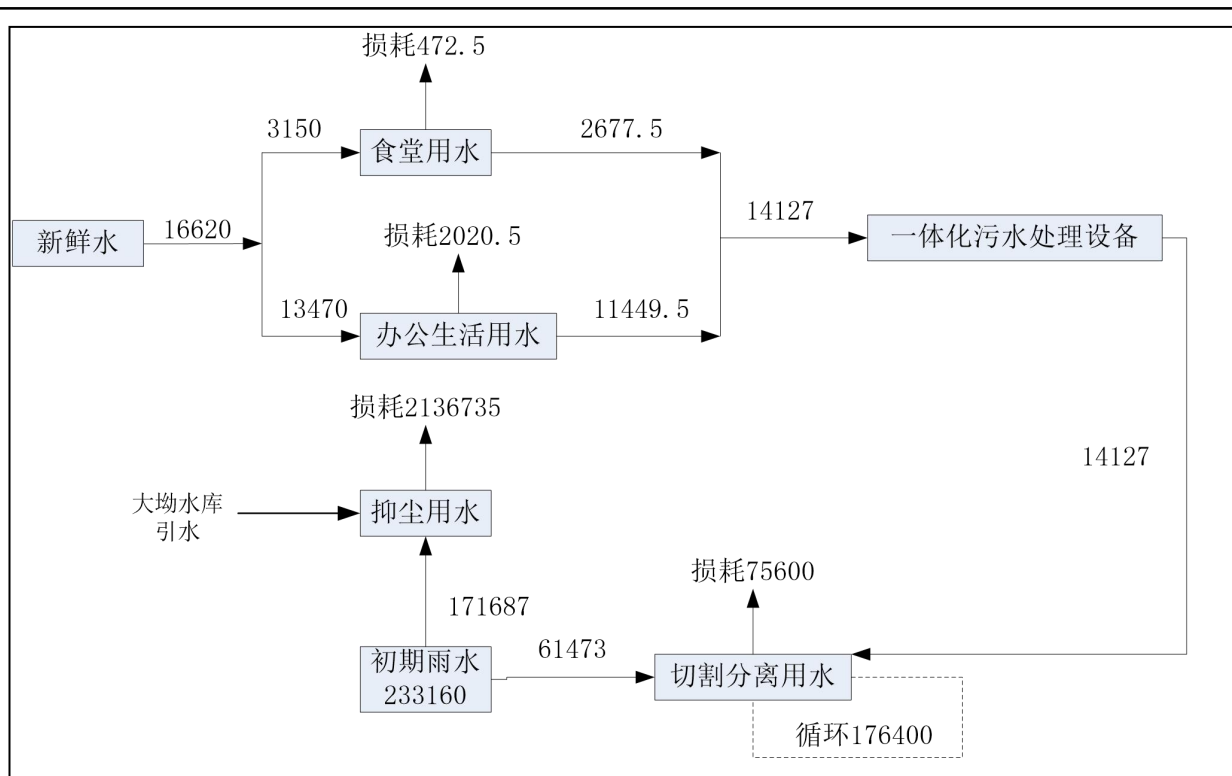
图 4-3 项目年水平衡图 单位：m³/a
