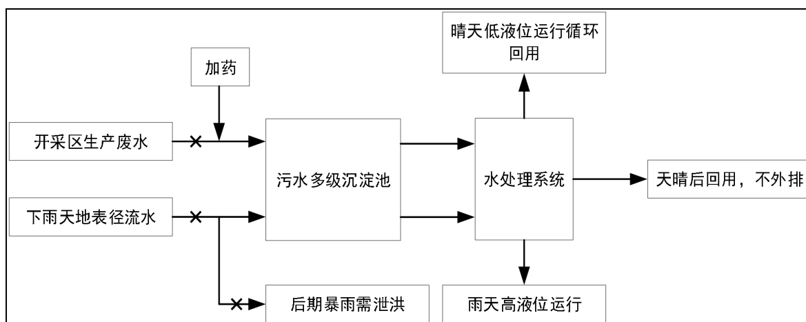
图 4-8 污、雨水收集池分流建设原则示意图
