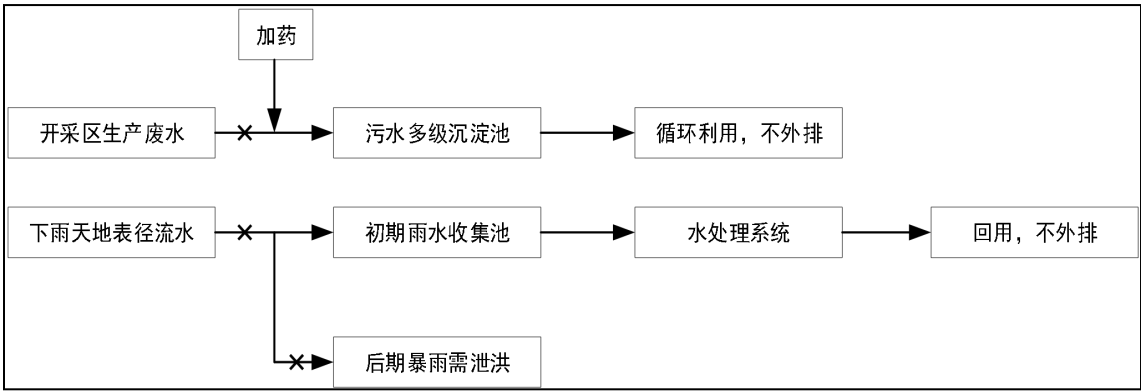
图 4-4 污、雨水收集池分流建设原则示意图
