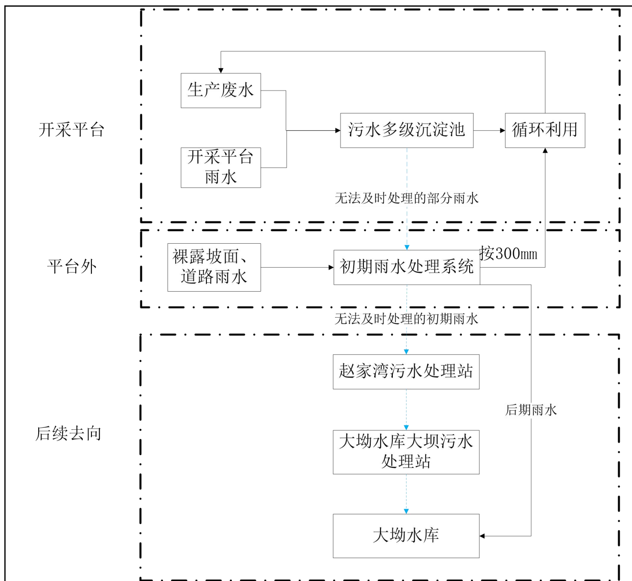
图 4-5 本项目排水流程示意图
