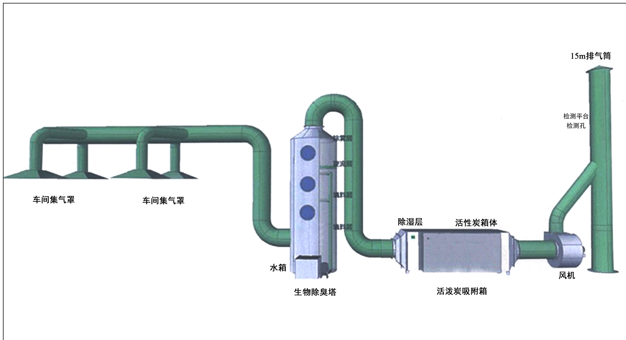
附图5 本项目恶臭废气收集处理工艺示意图
