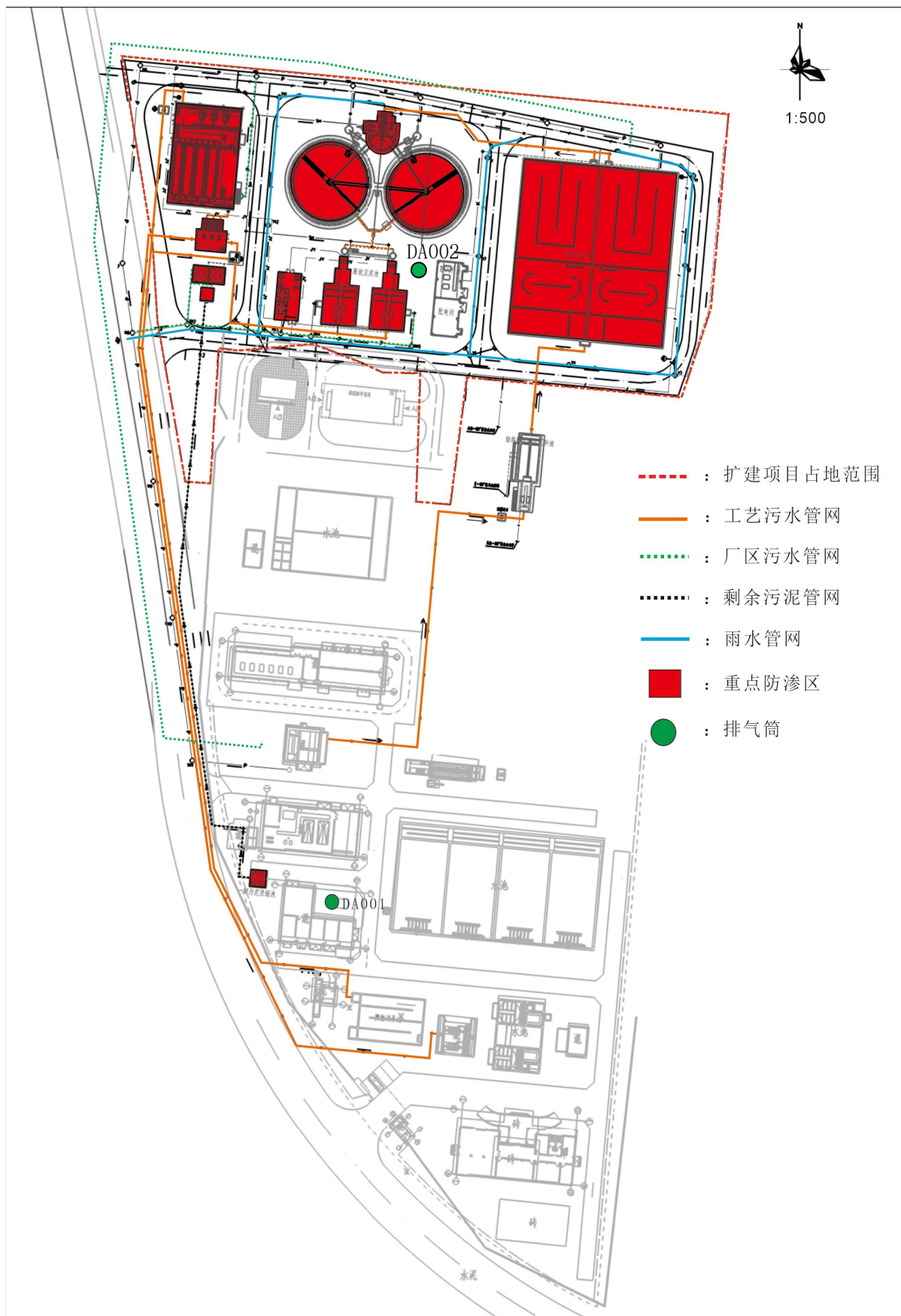
附图 4 扩建项目环保设施及雨污管网图
