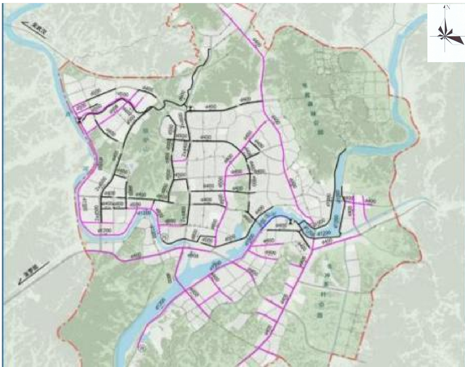
附图 7 英山县西汤河污水处理厂服务范围
