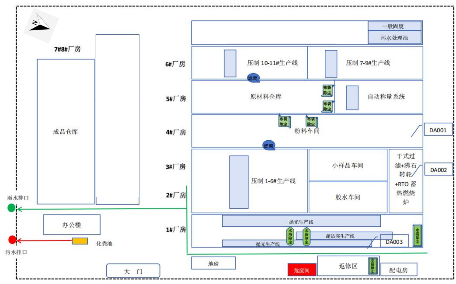
附图3 项目平面布置图及雨污管网图
